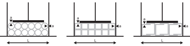
Het zagen van meerdere profielen tegelijk.
